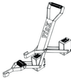
VVKRP krikgedeelte poot voor poot mecanisme avec alternative traction
